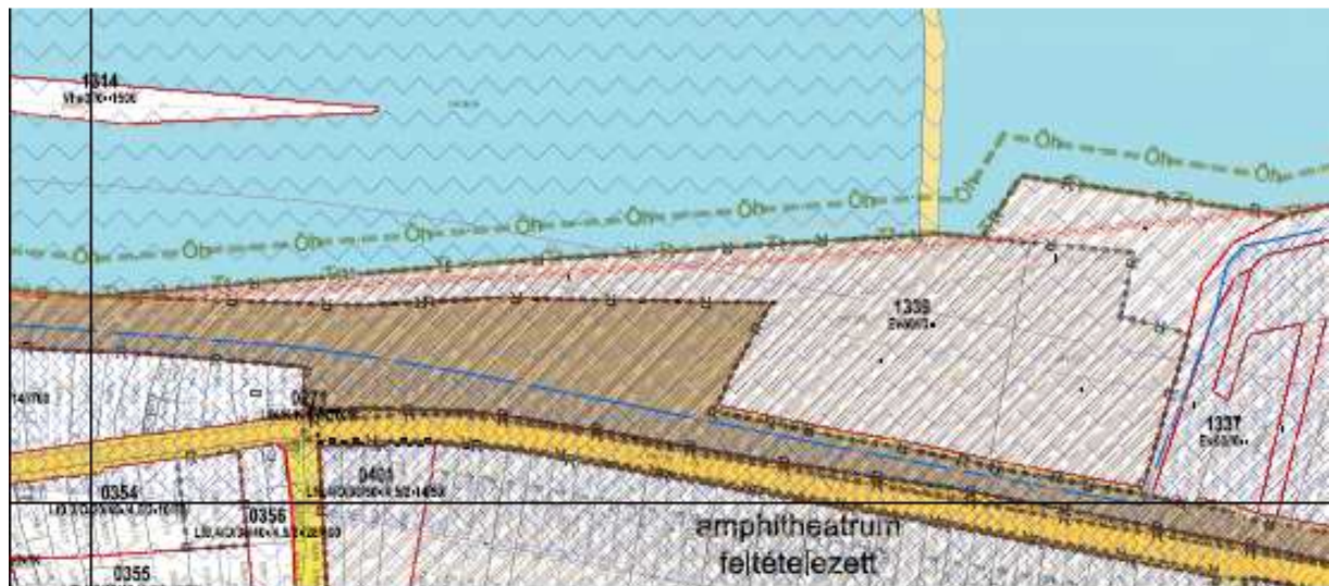
3. ábra: Részlet a szabályozási terv 74-314-23 szelvényéből. A tervezett látogatóközpont a barna színnel jelzett vasúti területnek az 1393-as övezettel szomszédos háromszög alakú részén fog elhelyezkedni a vasúti töltés és az új árvízvédelmi töltés között.
