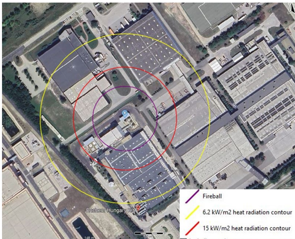
24. ábra - LEF.BLEVE esemény hatásövezetei
