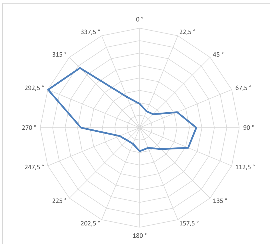
3. ábra: Komárom jellemző szélirányeloszlása. 7
