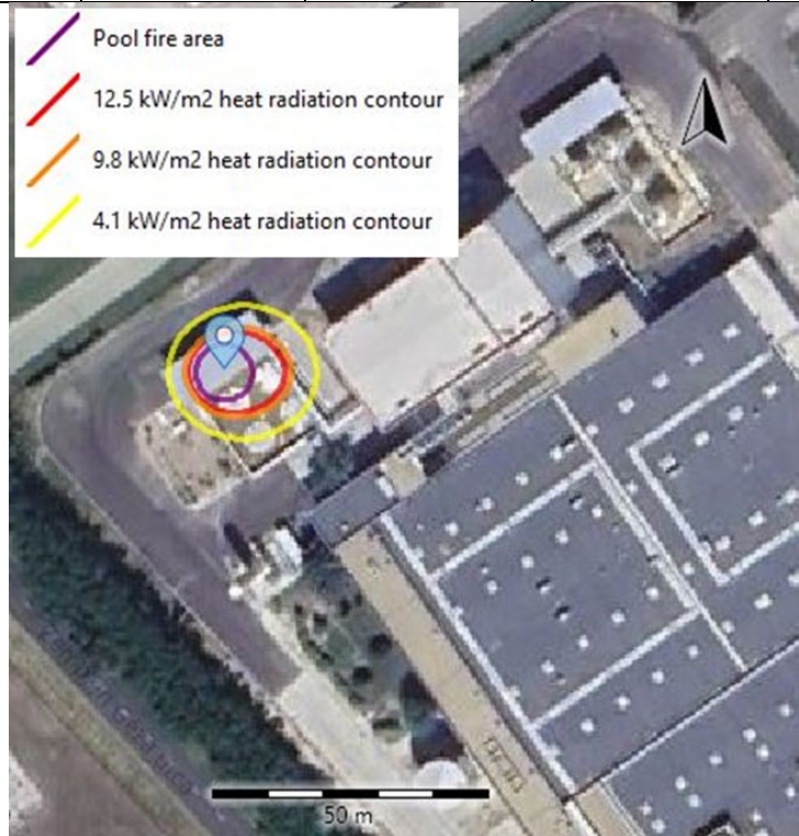
25. ábra: Befejtő - Tócsatűz
