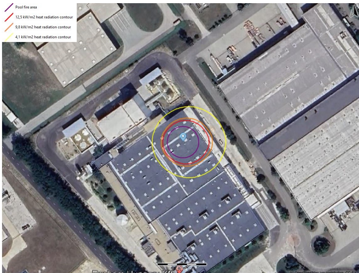
27. ábra: Elektrolit hordós tárolás - Tócsatűz
