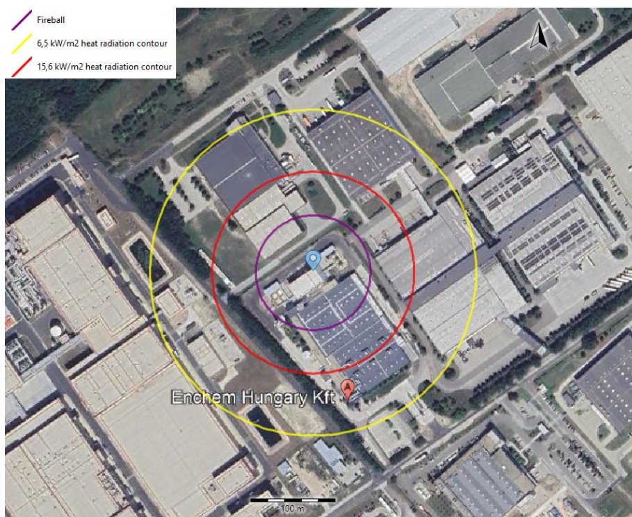
19. ábra – TP3.BLEVE esemény hatásövezetei (LiPF6 oldat belső tartály)
