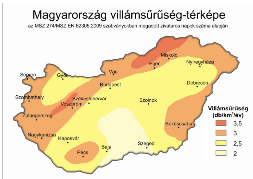
3. ábra: Magyarország villámsűrűség-térképe 12
